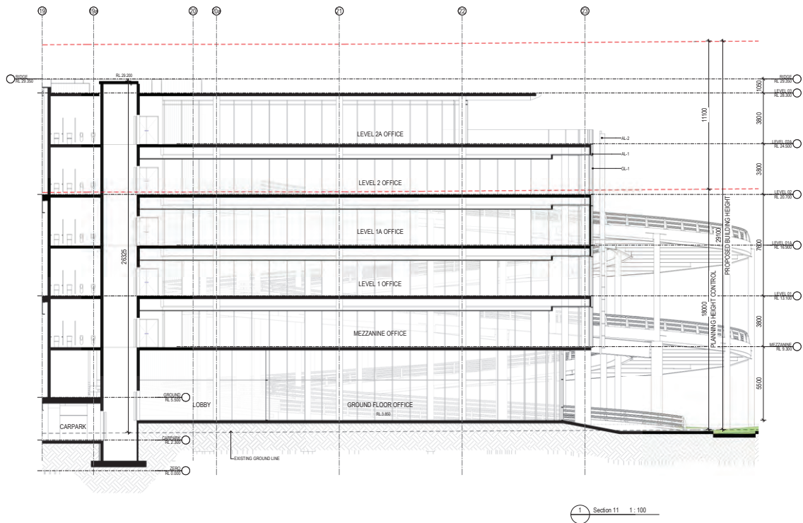
1 Section 11 1:100
